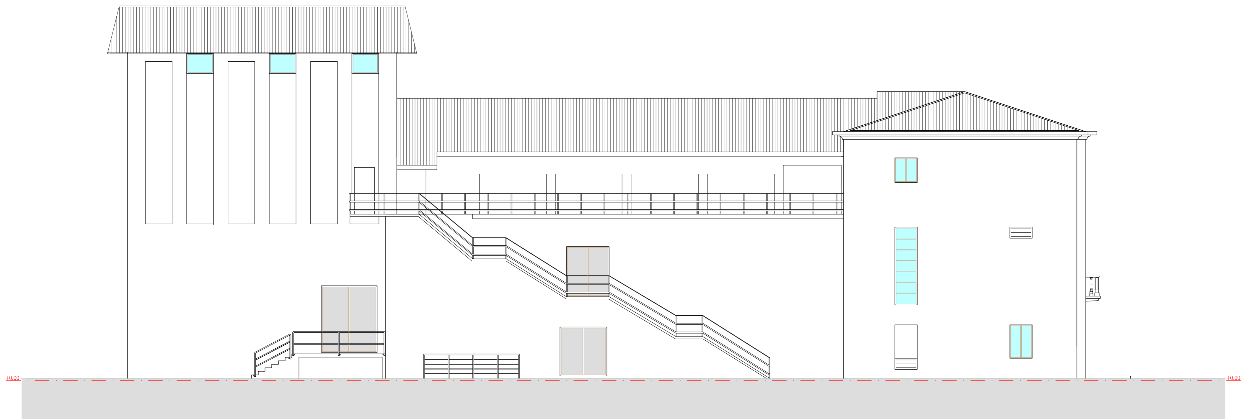
Prospetto nord
